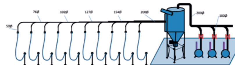
Schemat instalacji
